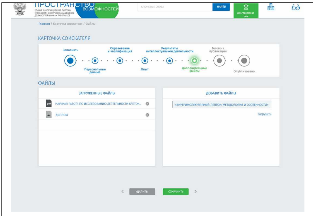
Рисунок 14 – Дополнительные файлы
